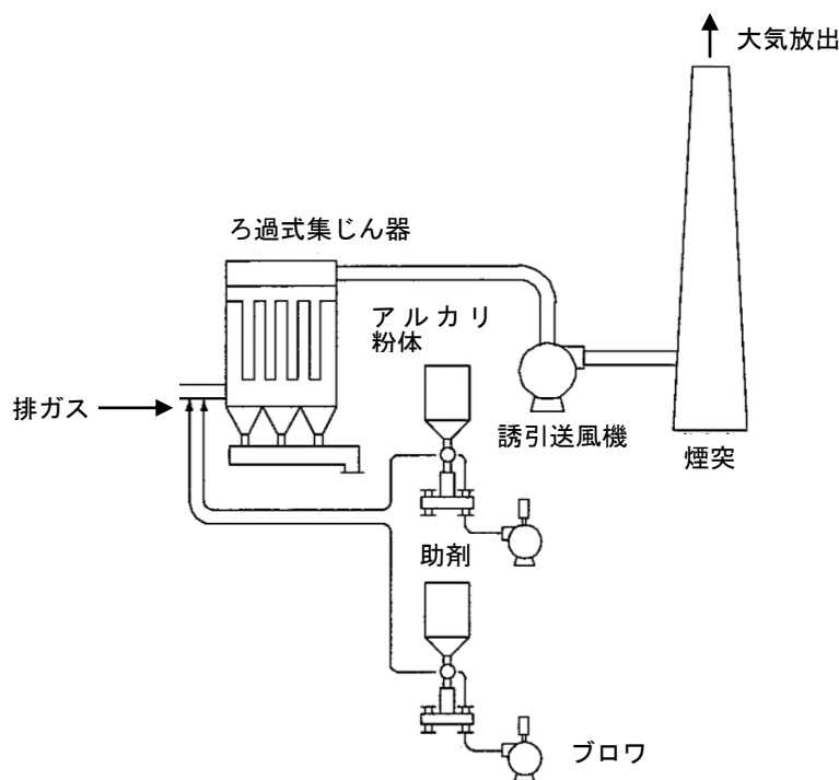
図 7-10 乾式有害ガス処理方式の除去フロー例
