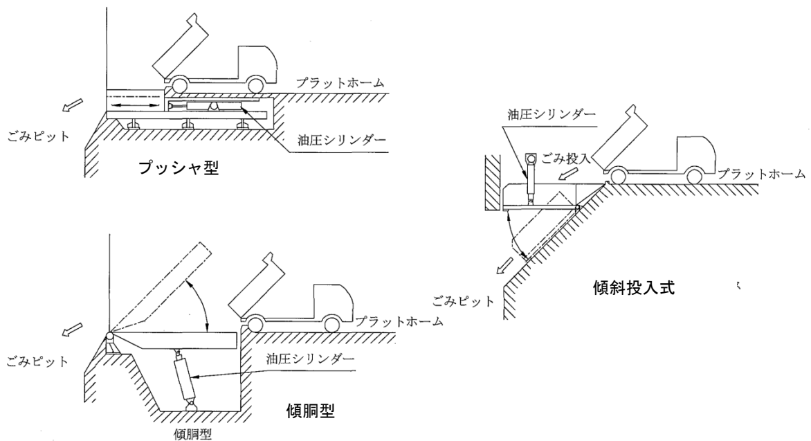
図 7-5 ダンプボックスの投入方式例
